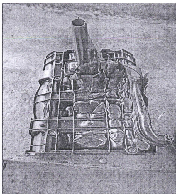
IMAGEM COM DETALHE DO TUBO DE ADMISSÃO DE ÓLEO DO MOTOR QUE FICOU TOTALMENTE DERRETIDO APÓS O SUPERAQUECIMENTO NO MOTOR
