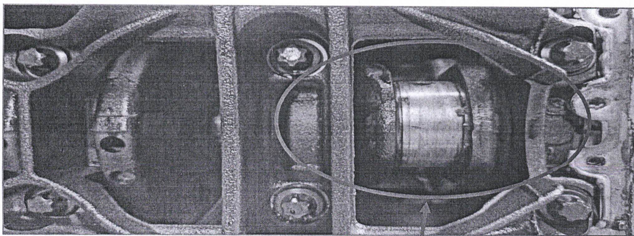
NESTA IMAGEM PODEMOS VER SINAIS CLAROS DO SUPERAQUECIMENTO OCORRIDO NO MOTOR, AS ALTÍSSIMAS TEMPERATURAS FIZERAM O MOTOR “GRIPAR”, MATERIAIS “COLARAM” LITERALMENTE
