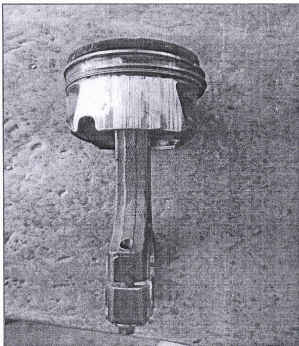
IMAGEM COM DETALHE DE UM DOS PISTÕES QUE FICOU COMPLETAMENTE DANIFICADO, SINAIS CLAROS DE RASPAGEM, ANÉIS GRIPADOS
